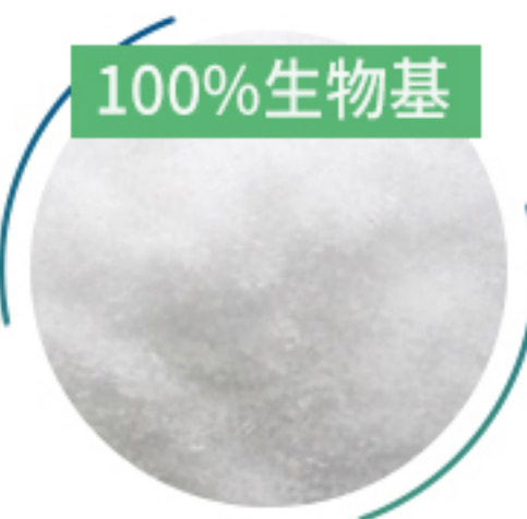
氨基11酸
